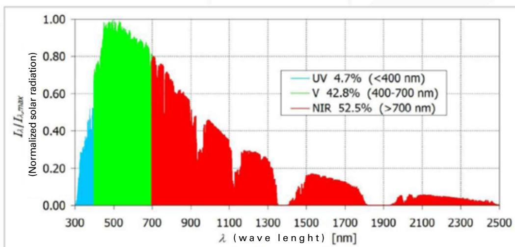
Figura 1.1 Spettro normalizzato della radiazione solare alla superfici terrestri (dati dall'ASTM Standard G173). / Figure 1.1 Normalized solar radiation spectrum at the Earth's surface (data from ASTM Standard G173).
